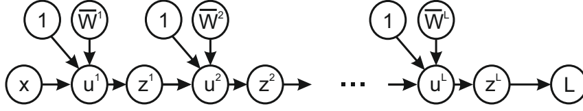
Рис. 2: Граф вычислений для автокодировщика
