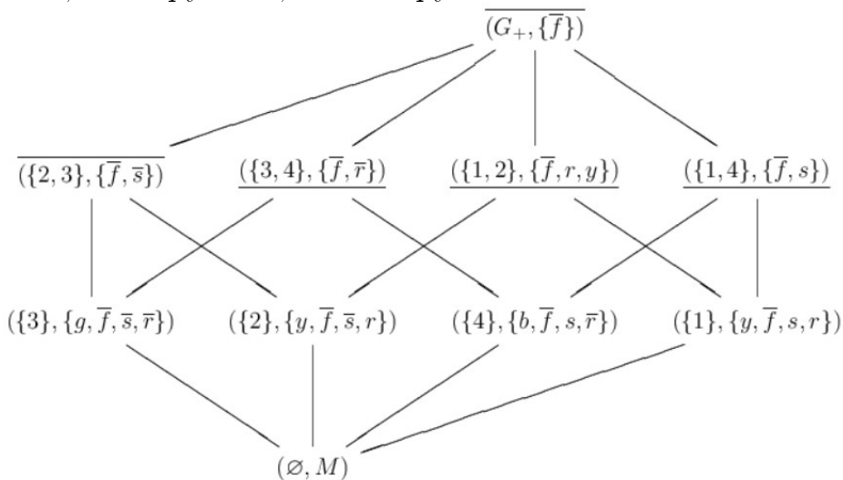
Рис. 4.14. Решётка \mathfrak{B}(K_+)
