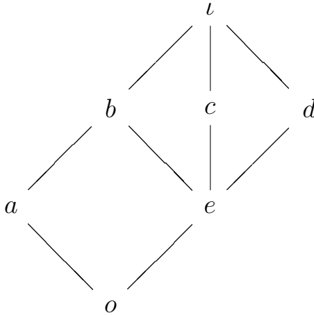
Рис. 4.13. Решётка с относительными дополнениями
