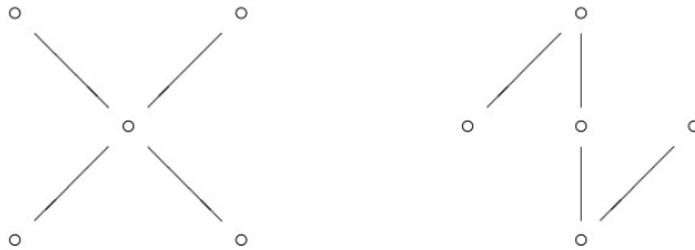
Рис. 3.13. 5-элементные самодвойственные ч.у. множества
