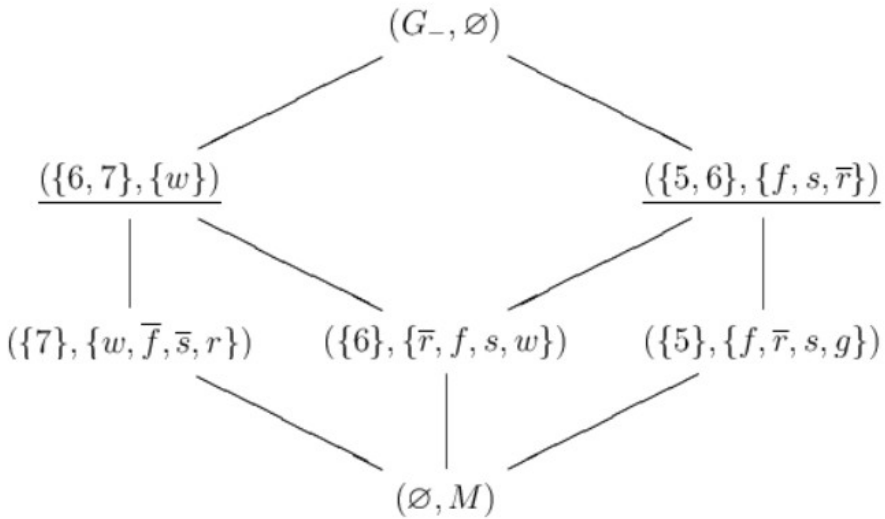
Рис. 4.15. Решётка \mathfrak{B}(K_-)
