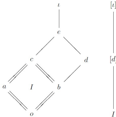
Рис. 4.12. Множество I = \{o, a, b, c\} — идеал решётки
