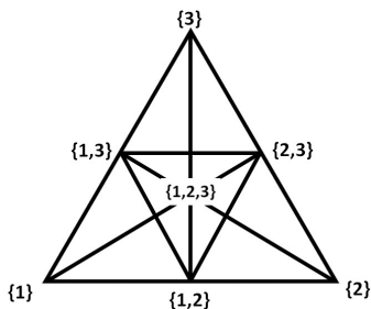
Рис. 2.2. Графовое представление симплекса S^3
