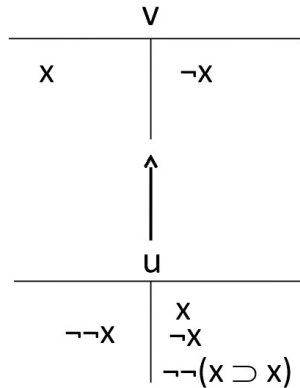
Рис. 3.23. Контрмодель для \neg\neg x \supset x
