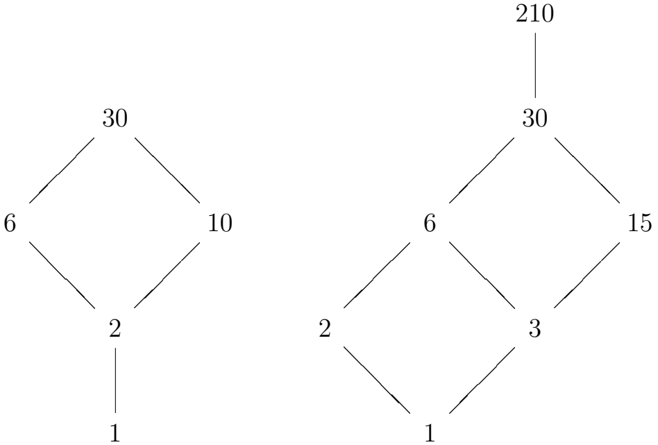
Рис. 4.11. Вложение L \hookrightarrow \langle \mathbb{N}, | \rangle
