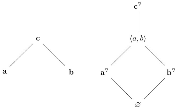
Рис. 4.9. Z_3 , множество \text{Irr } J(Z_3) выделено
