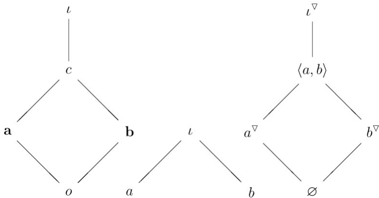
Рис. 4.10. Иллюстрация ФТКДР: L , Irr L и J(Irr L)
