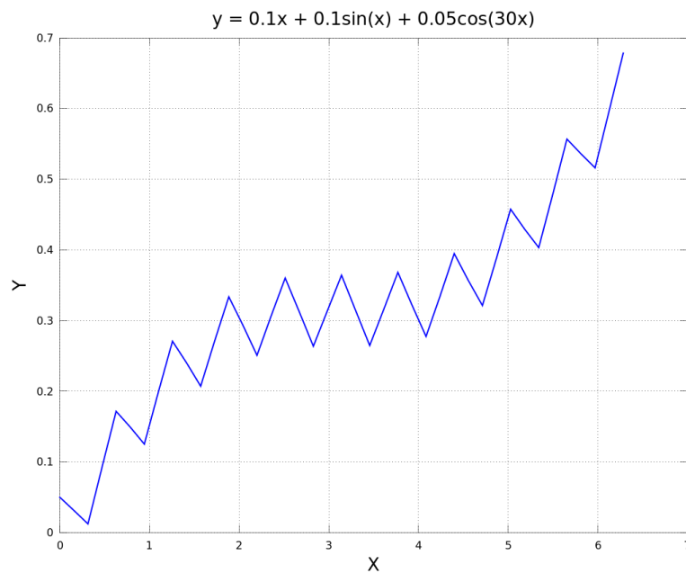
Рис. 13. График функции y = 0.1x + 0.1\sin(x) + 0.05\cos(30x) .
