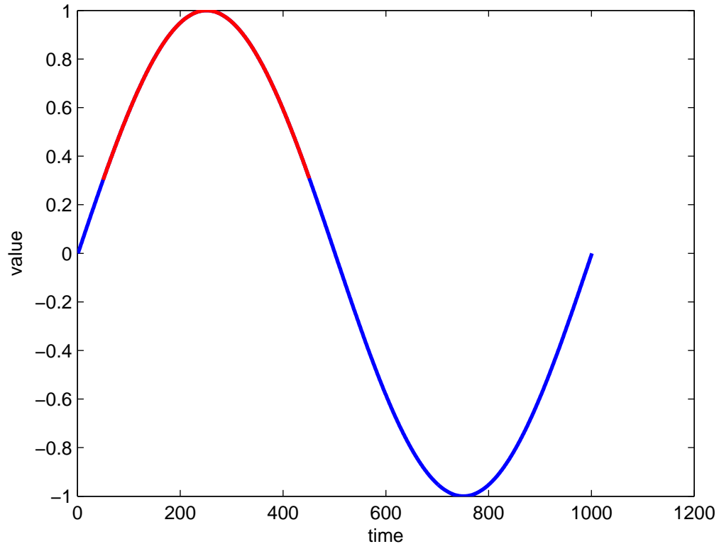
Рис. 3. Последовательность Q и подпоследовательность Q' в ней.
