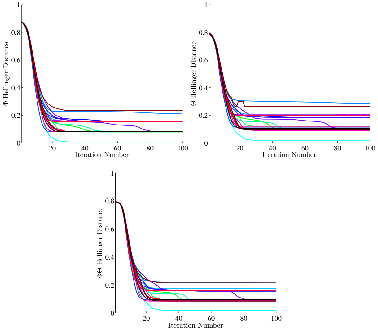
Рис. 3: Сходимость расстояния Хеллингера для матриц \Phi , \Theta и \Phi\Theta соответственно (модельные данные, метод [10])
