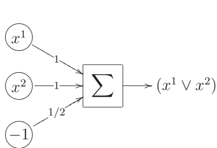
Рис. 18. Однослойный перцептрон, реализующий операцию ИЛИ.
