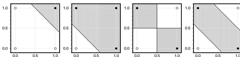
Рис. 20. Перцептронная реализация элементарных логических функций. Слева направо: И, ИЛИ, XOR с помощью добавления признака x^1x^2 , XOR с помощью двухслойной сети.
