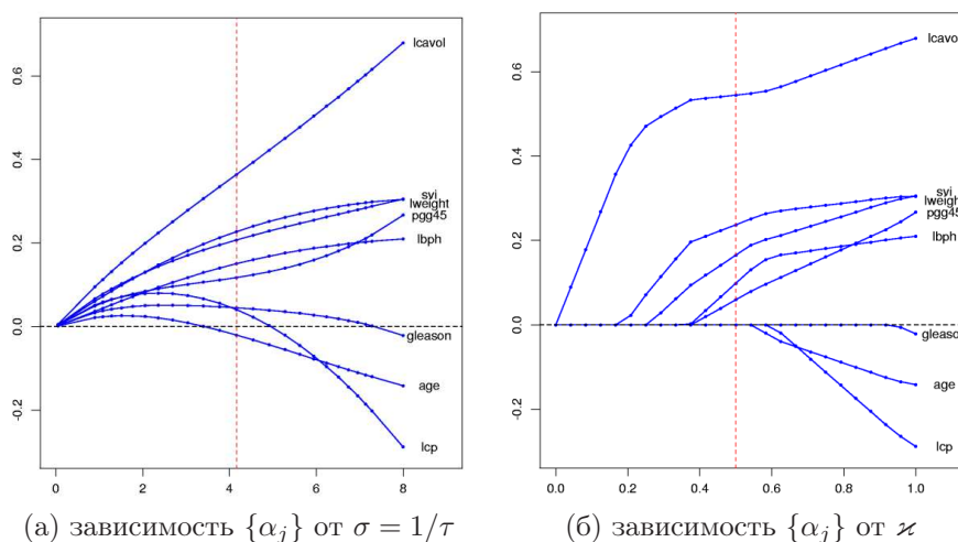
Рис. 16. Зависимость коэффициентов линейной модели от параметра \sigma = 1/\tau для гребневой регрессии и от параметра \lambda для лассо Тибширани, по реальным данным задачи UCI.cancer [44].
