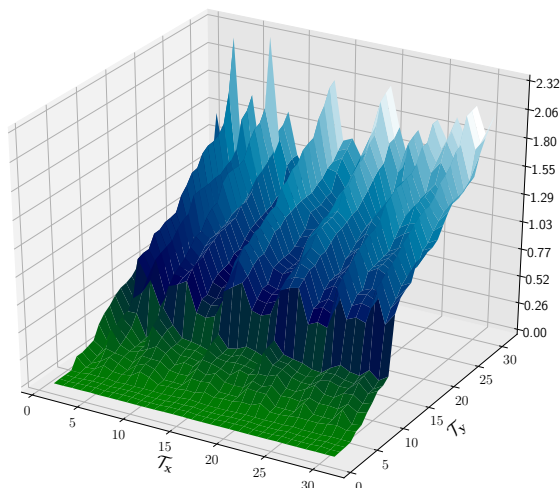
Рис. 14: Отношение расстояния между ближайшими соседями ряда x к расстоянию между соседями ряда y . Ближайшие соседи определяются по ряду x
