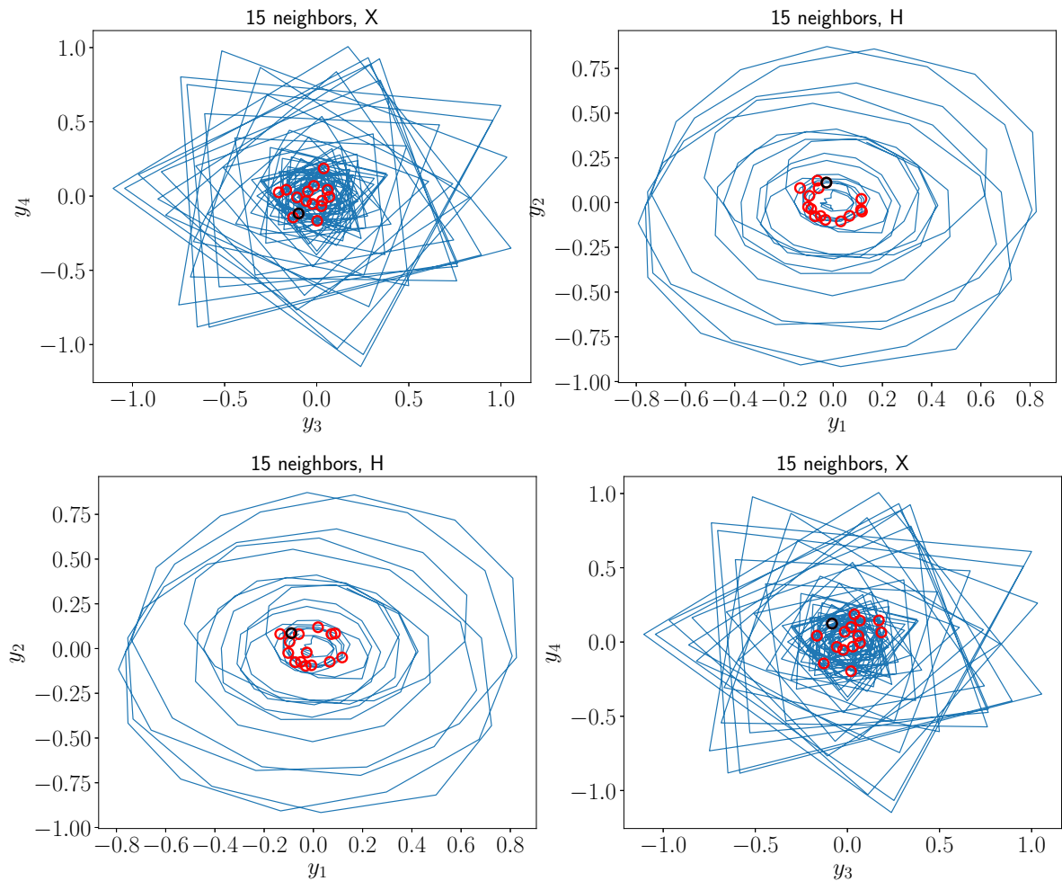
Рис. 19: Связи между рядами x и h
