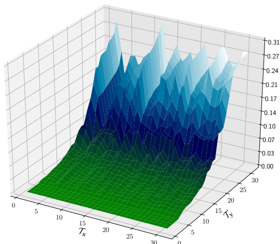
Рис. 15: Отношение расстояния между ближайшими соседями ряда y к расстоянию между соседями ряда x . Ближайшие соседи определяются по ряду x
